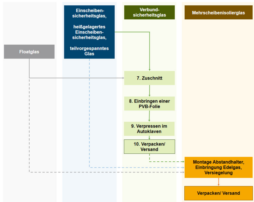
Abbildung 1 Herstellungsprozess
