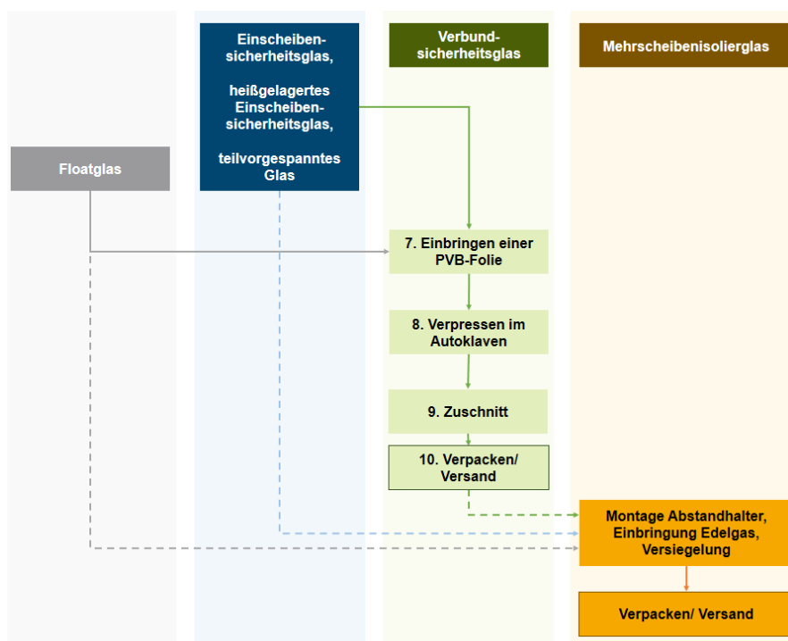
Abbildung 1 Herstellungsprozess
