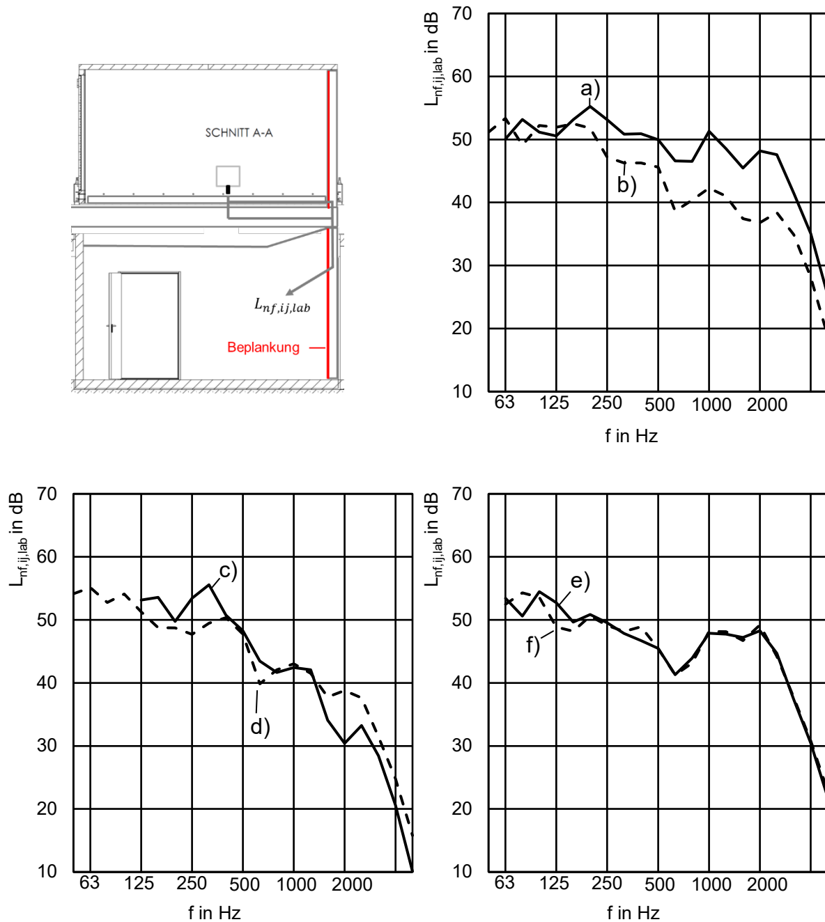
Abbildung 8 Norm-Trittschallpegel flankierender Bauteile L_{nf,ij,lab} für eine Holzbalkendecke mit Zementestrich auf 30 mm Mineralfaser-Trittschalldämmplatten. Flankierende Holztafelbauwand mit unterschiedlichen Beplankungen. Bezugsgrößen: |S_{i,lab}| = |h_{ij,lab}| a) 12 mm OSB: L_{nf,ij,lab,w} = 53 dB b) 12 mm OSB + 12,5 mm GK, f_c \approx 2500 Hz: L_{nf,ij,lab,w} = 47 dB c) 2 × 12,5 mm GKF, f_c \approx 2500 Hz: L_{nf,ij,lab,w} = 47 dB d) 2 × 18 mm GF, f_c \approx 2000 - 2500 Hz: L_{nf,ij,lab,w} = 47 dB e) 1 × 18 mm GKF, f_c \approx 1600 - 2000 Hz: L_{nf,ij,lab,w} = 51 dB f) 2 × 18 mm GKF, f_c \approx 1600 - 2000 Hz: L_{nf,ij,lab,w} = 51 dB
