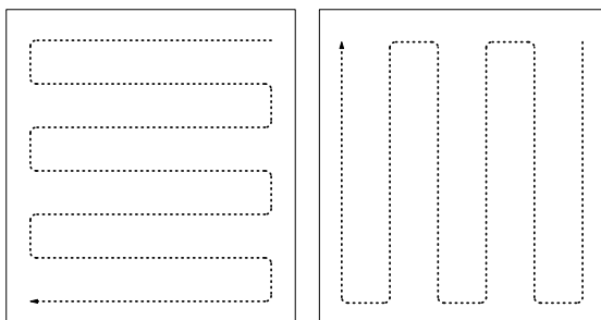
Abbildung 2 Abtastschema für die horizontale und vertikale Abtastung
