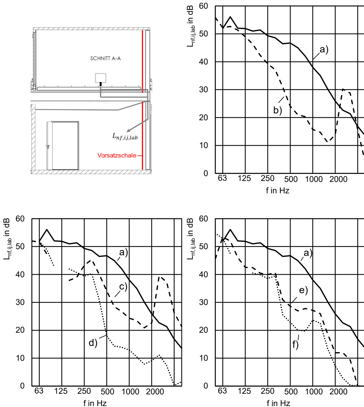
Abbildung 10 Norm-Trittschallpegel flankierender Bauteile L_{nf,ij,lab} für eine Massivholzdecke mit 60 mm Splitt und Zementstrich auf 30 mm Mineralfaser-Trittschalldämmplatten. Flankierende Massivholzwand (80 mm CLT) mit unterschiedlichen Vorsatzschalen. Bezugsgrößen: |S_{i,lab}| = |I_{ij,lab}| a) 80 mm CLT: L_{nf,ij,lab,w} = 45 dB b) 80 mm CLT + 27 mm Federschiene mit 30 MW + 12,5 mm GK: L_{nf,ij,lab,w} = 41 dB c) 80 mm CLT + 40 mm Lattung + 2 × 12,5 mm GK: L_{nf,ij,lab,w} = 41 dB d) 80 mm CLT + 60 mm entkoppelte Lattung + 12,5 mm GK: L_{nf,ij,lab,w} = 33 dB e) 80 mm CLT + 10 mm Luft + 75 mm CW + 2 × 12,5 mm GK: L_{nf,ij,lab,w} = 35 dB f) 80 mm CLT + 10 mm Luft + 75 mm CW + 2 × 12,5 mm GK, mit gleitendem Deckenanschluss an der Massivholzdecke: L_{nf,ij,lab,w} = 30 dB
