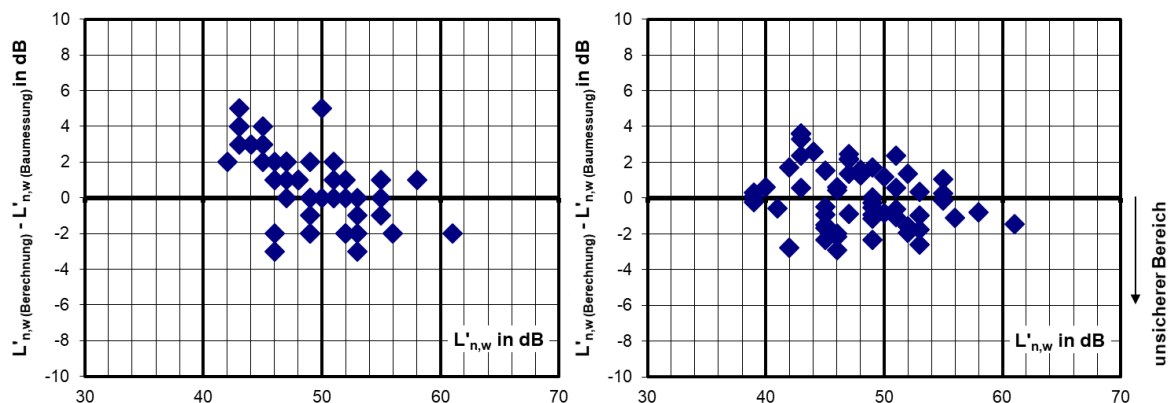
Abbildung 23 Validierung des Berechnungsmodell für 63 Baumessungen in Holzbauten.
