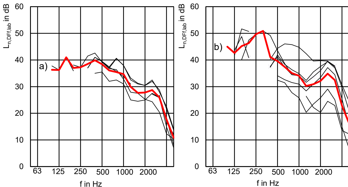
Abbildung 16 Norm-Flanken-Trittschallpegel L_{n,Df,lab} für eine Holzbalkendecke mit unterschiedlichen Estrichaufbauten. Flankierende Holztafelbauwand mit OSB und GK-Beplankung. Bezugsgrößen: |S_{i,lab}| = |I_{lab}|
