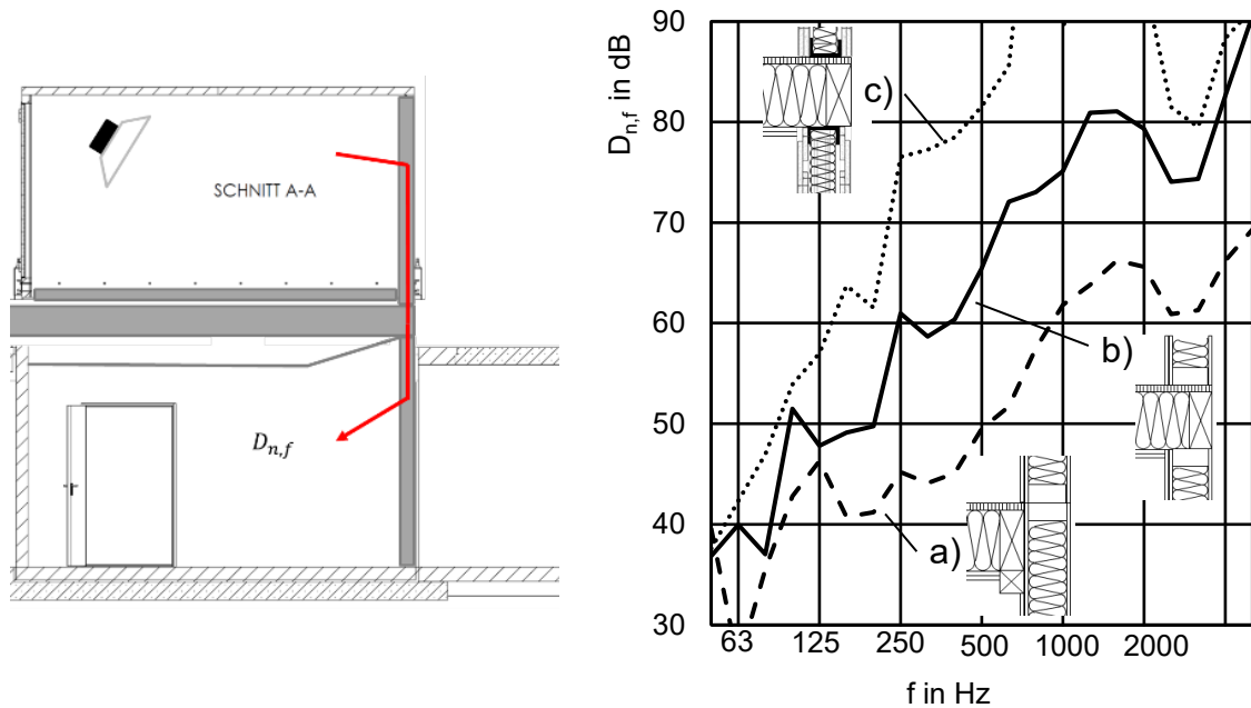
Abbildung 17 Norm-Flankenschallpegeldifferenz D_{n,f} für unterschiedliche flankierende Wände und Deckenanschlüsse einer Holzbalkendecke. Bezugsgrößen: S_0 = 10 \text{ m}^2 ; l_0 = 4,50 \text{ m} a) Holztafelbauwand durchlaufend, aber auf Deckenhöhe gestoßen, Decke vorgehängt (quasi-ballon-framing) Beplankung mit 12 mm OSB + 12,5 mm GK: D_{n,f,w} = 54 \text{ dB} b) Holztafelbauwand durch die Decke vollständig unterbrochen (platform-framing) Beplankung mit 12 mm OSB + 12,5 mm GK: D_{n,f,w} = 67 \text{ dB} c) Metallständerwand (C-Profil) mit gleitendem Deckenanschluss. Beplankung mit 2 \times 12,5 \text{ mm GK} : D_{n,f,w} = 79 \text{ dB}
