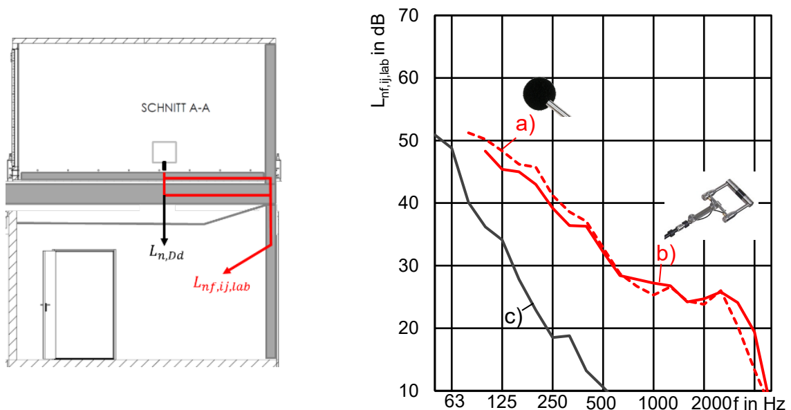
Abbildung 5 Norm-Trittschallpegel flankierender Bauteile L_{nf,ij,lab} für eine Massivholzdecke mit 60 mm Splitt und Zementestrich auf 30 mm Mineralfaser-Trittschalldämmplatten. Flankierende Holztafelbauwand mit OSB und GK-Beplankung. Bezugsgrößen:
