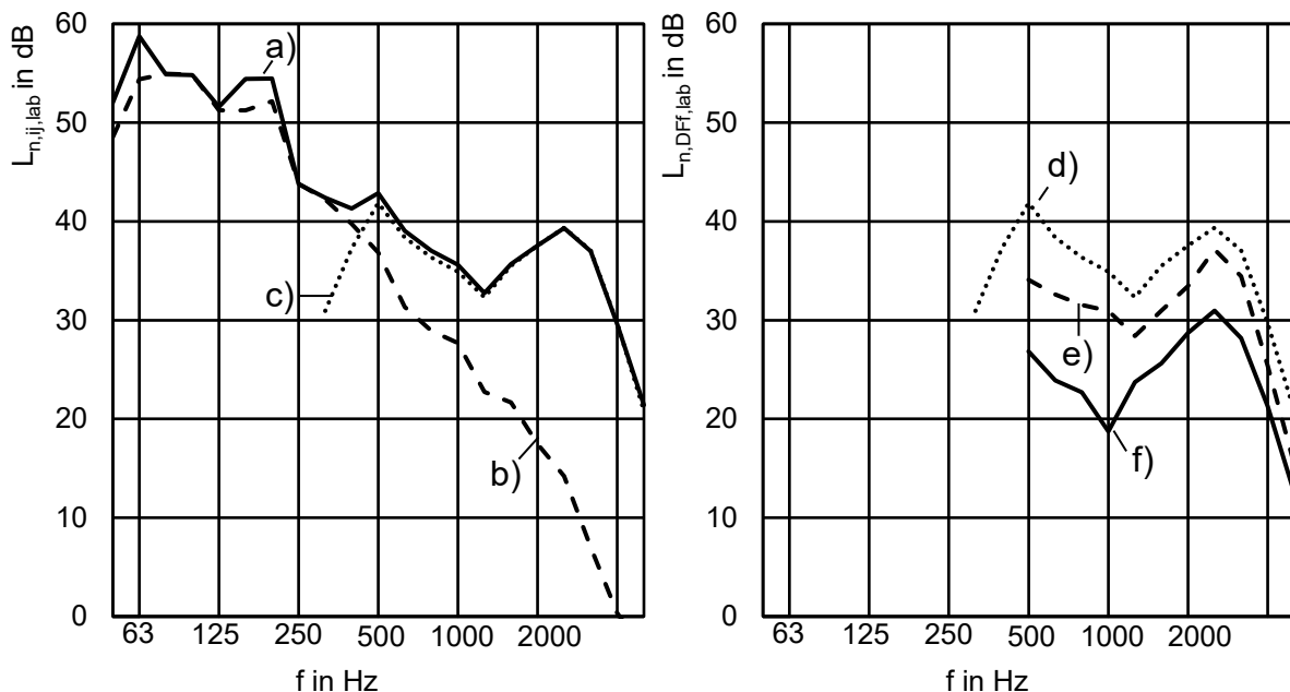
Abbildung 14 Norm-Trittschallpegel flankierender Bauteile für eine Holzbalkendecke mit 60 mm Splitt und Zementestrich auf 30 mm Holzfaser-Trittschalldämmplatten. Flankierende Holztafelbauwand mit OSB und GK-Beplankung.
