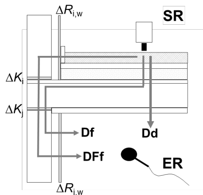
Abbildung 22 Anordnung von Vorsatzschalen und Elastomerlagern
