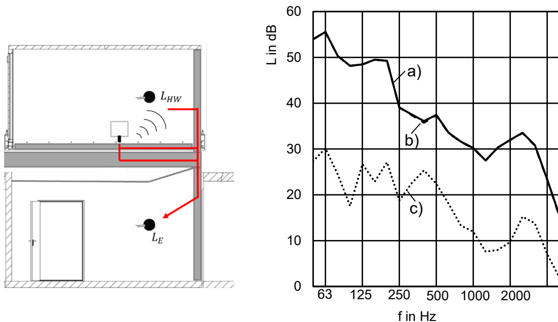
Abbildung 15 Pegelmessungen für die Luftschallkorrektur nach DIN 4109-4. Decken- und Wand-aufbau wie in Abbildung 14. S_{i,lab} = 20 \text{ m}^2 , h_{ij,lab} = 4,0 \text{ m}
