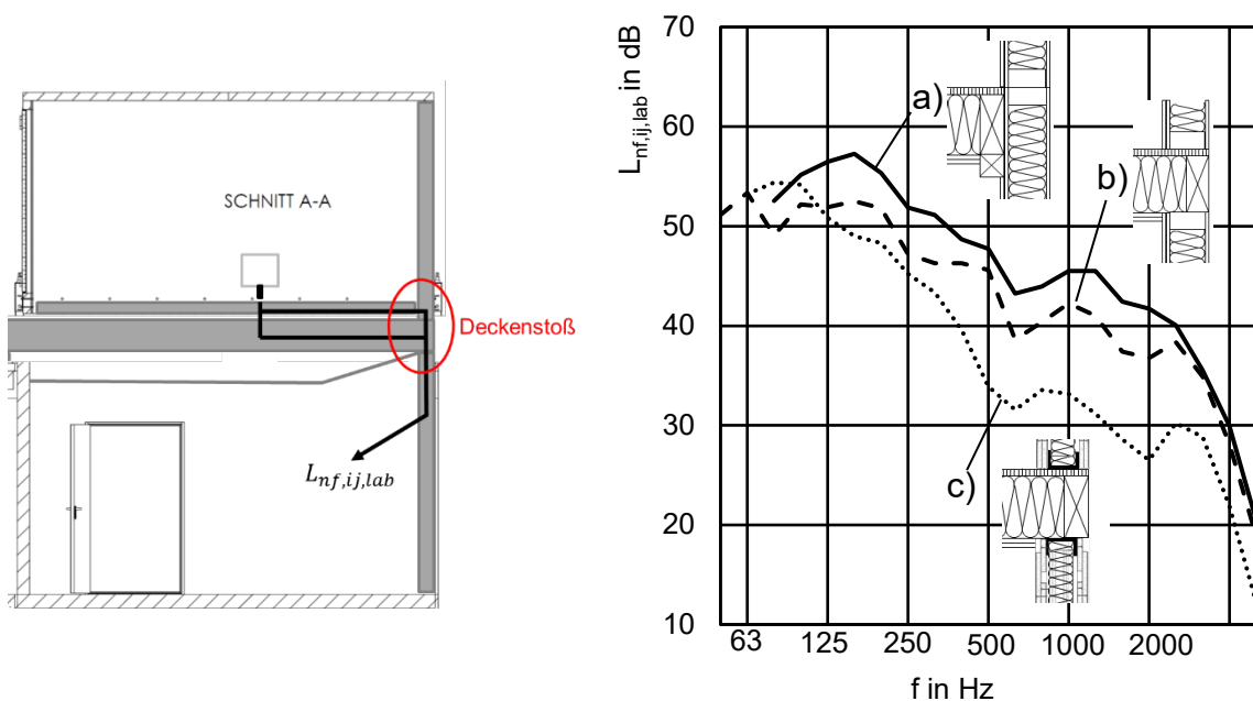
Abbildung 11 Norm-Trittschallpegel flankierender Bauteile L_{nf,ij,lab} für eine Holz balkendecke mit Zementestrich auf 30 mm Mineralfaser-Trittschalldämmplatten. Flankierende Wände und Deckenstoß unterschiedlich ausgeführt. Bezugsgrößen: |S_{i,lab}| = |I_{ij,lab}| a) Holztafelbauwand durchlaufend, aber auf Deckenhöhe gestoßen, Decke vorgehängt (quasi-ballon-framing) Beplankung mit 12 mm OSB + 12,5 mm GK: L_{nf,ij,lab,w} = 50 dB b) Holztafelbauwand durch die Decke vollständig unterbrochen (platform-framing) Beplankung mit 12 mm OSB + 12,5 mm GK: L_{nf,ij,lab,w} = 47 dB c) Metallständerwand (C-Profil) mit gleitendem Deckenanschluss. Beplankung mit 2 × 12,5 mm GK: L_{nf,ij,lab,w} = 43 dB
