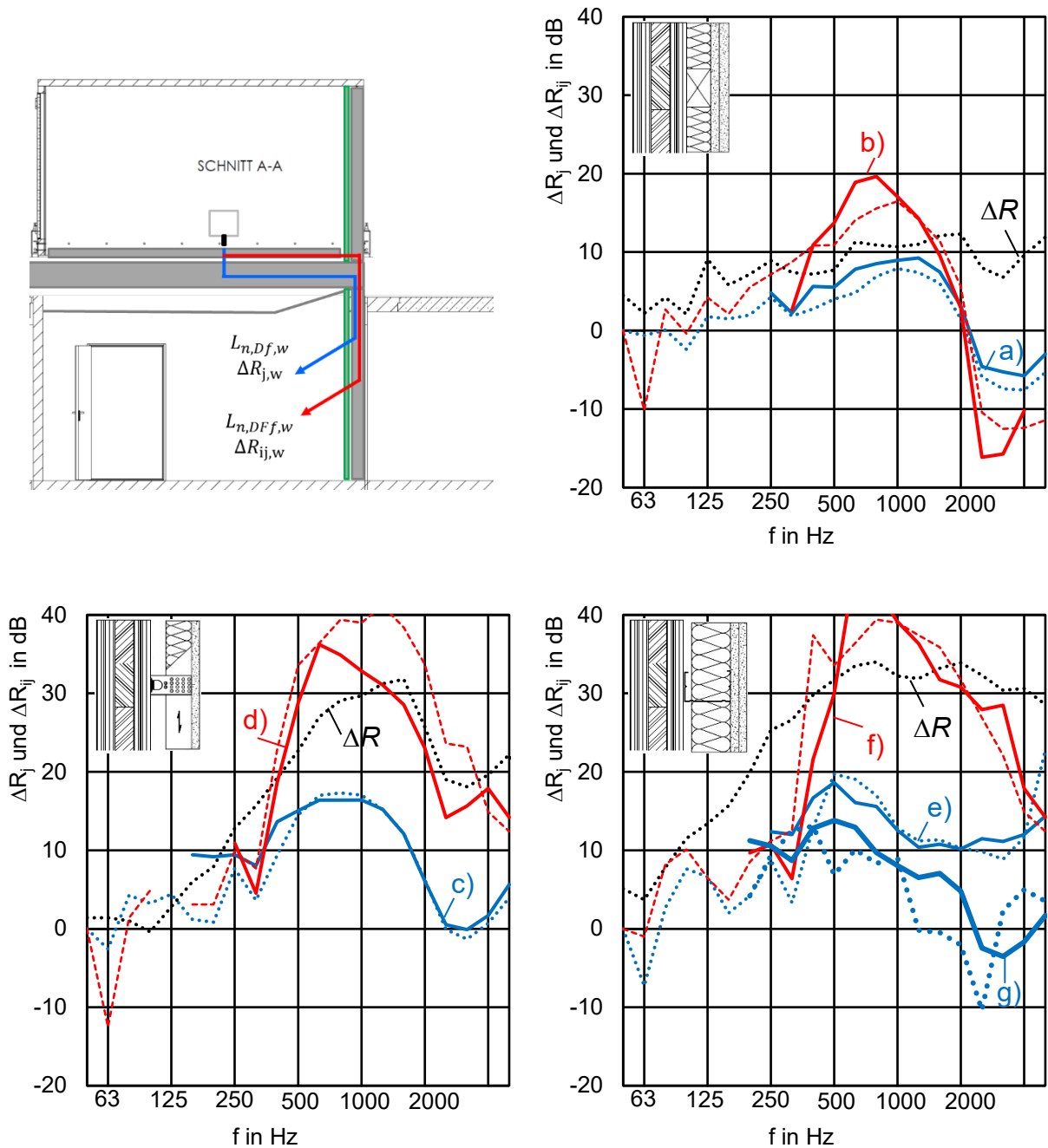
Abbildung 20 Verbesserung durch unterschiedliche Vorsatzschalen bei Trittschallanregung (durchgezogene Linien) und Luftschallanregung (gepunktete Linien) für die Übertragungswege Df und DFf (Maße in mm):
