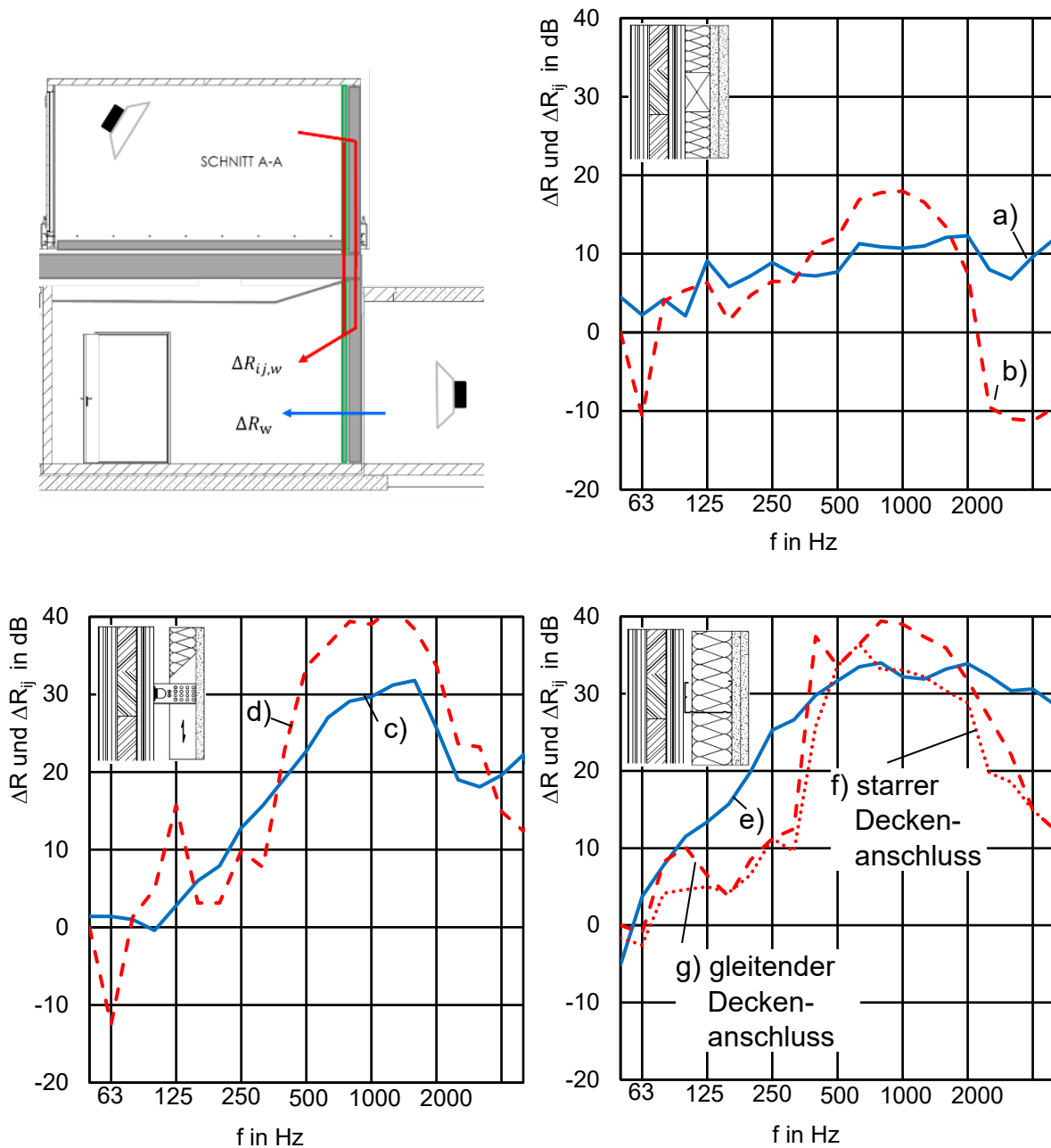
Abbildung 19 Verbesserung der Schalldämmung \Delta R und der Flankendämmung \Delta R_{ij} von Massivholzwänden durch unterschiedliche Vorsatzschalen (Maße in mm):
