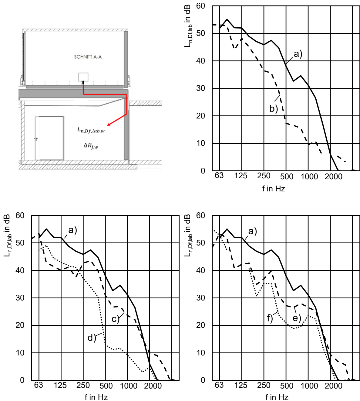
Abbildung 13 Norm-Flanken-Trittschallpegel L_{n,Df,lab,w} für eine Massivholzdecke mit 60 mm Splitt und Zementestrich auf 30 mm Mineralfaser-Trittschalldämmplatten. Flankierende Massivholzwand (80 mm CLT) mit unterschiedlichen Vorsatzschalen. Bezugsgrößen: |S_{i,lab}| = |I_{ij,lab}| a) 80 mm CLT: L_{n,Df,lab,w} = 42 dB b) 80 mm CLT + 27 mm Federschiene mit 30 MW + 12,5 mm GK: L_{n,Df,lab,w} = 35 dB c) 80 mm CLT + 40 mm Lattung + 2 × 12,5 mm GK: L_{n,Df,lab,w} = 35 dB d) 80 mm CLT + 60 mm entkoppelte Lattung + 12,5 mm GK: L_{n,Df,lab,w} = 32 dB e) 80 mm CLT + 10 mm Luft + 75 mm CW + 2 × 12,5 mm GK: L_{n,Df,lab,w} = 33 dB f) 80 mm CLT + 10 mm Luft + 75 mm CW + 2 × 12,5 mm GK, mit gleitendem Deckenanschluss an der Massivholzdecke: L_{n,Df,lab,w} = 27 dB
