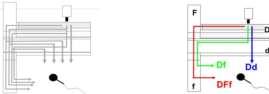
Abbildung 21 Flankierende Trittschallübertragung. Links: Mögliche Übertragungswege über die einzelnen Bauteilschichten. Rechts: Für die Berechnung berücksichtigte Übertragungswege.
