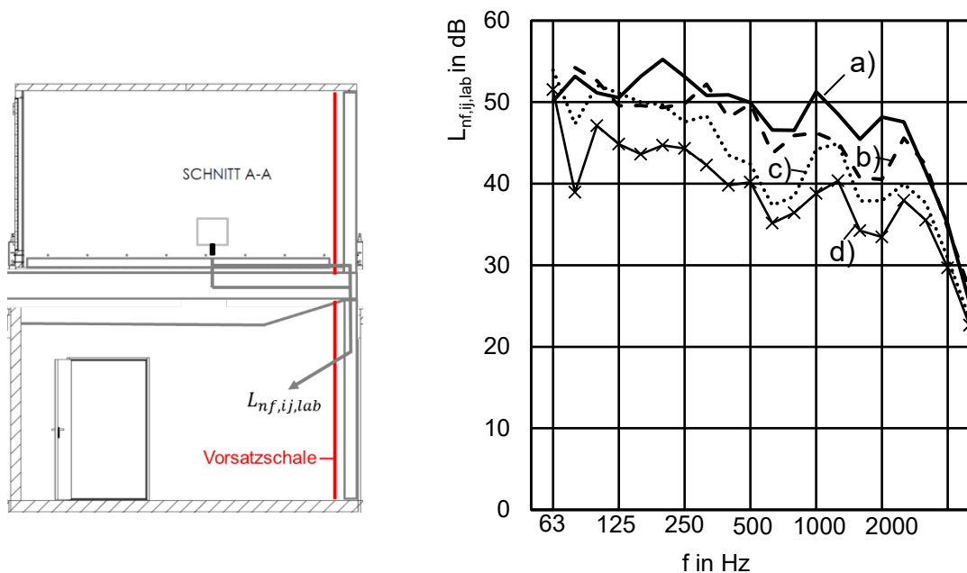
Abbildung 9 Norm-Trittschallpegel flankierender Bauteile L_{nf,ij,lab} für eine Holzbalkendecke mit Zementestrich auf 30 mm Mineralfaser-Trittschalldämmplatten. Flankierende Holztafelbauwand mit unterschiedlichen Vorsatzschalen. Bezugsgrößen: |S_{i,lab}| = |I_{ij,lab}| a) 12 mm OSB: L_{nf,ij,lab,w} = 53 dB b) 12 mm OSB + 40 mm Lattung + 12,5 mm GK: L_{nf,ij,lab,w} = 50 dB c) 12 mm OSB + 60 mm entkoppelte Lattung + 12,5 mm GK: L_{nf,ij,lab,w} = 47 dB d) 12 mm OSB + 10 mm Luft + 75 mm CW + 2 × 12,5 mm GK: L_{nf,ij,lab,w} = 43 dB
