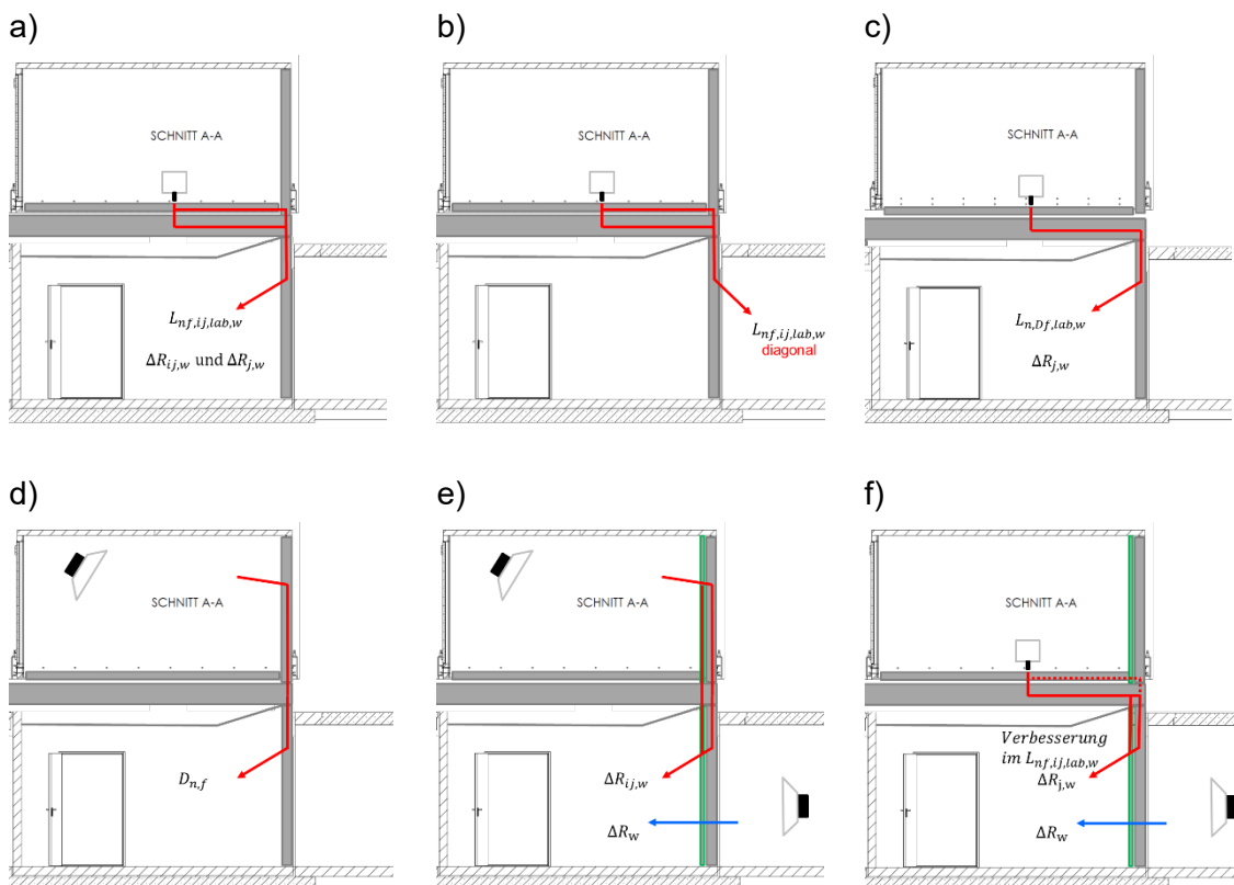
Abbildung 4 Untersuchte Flankenübertragungswege bei Luft und Trittschallanregung
