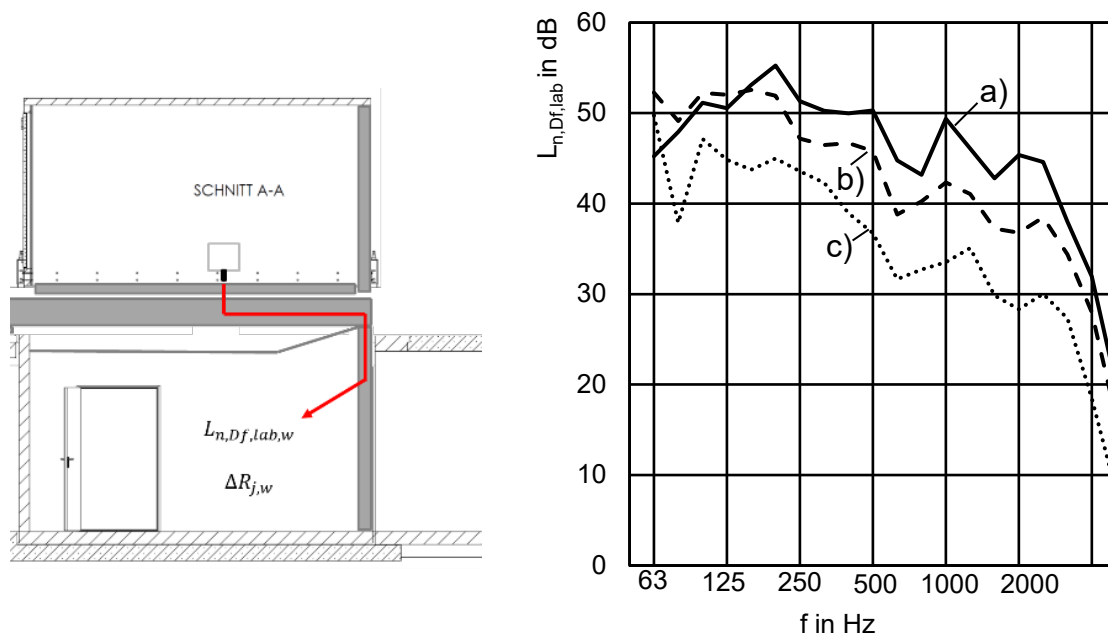
Abbildung 12 Norm-Flanken-Trittschallpegel L_{n,Df,lab,w} für eine Holzbalkendecke mit Zementestrich auf 30 mm Mineralfaser-Trittschalldämmplatten. Flankierende Holztafelbauwand mit unterschiedlichen Beplankungen und Vorsatzschalen.
