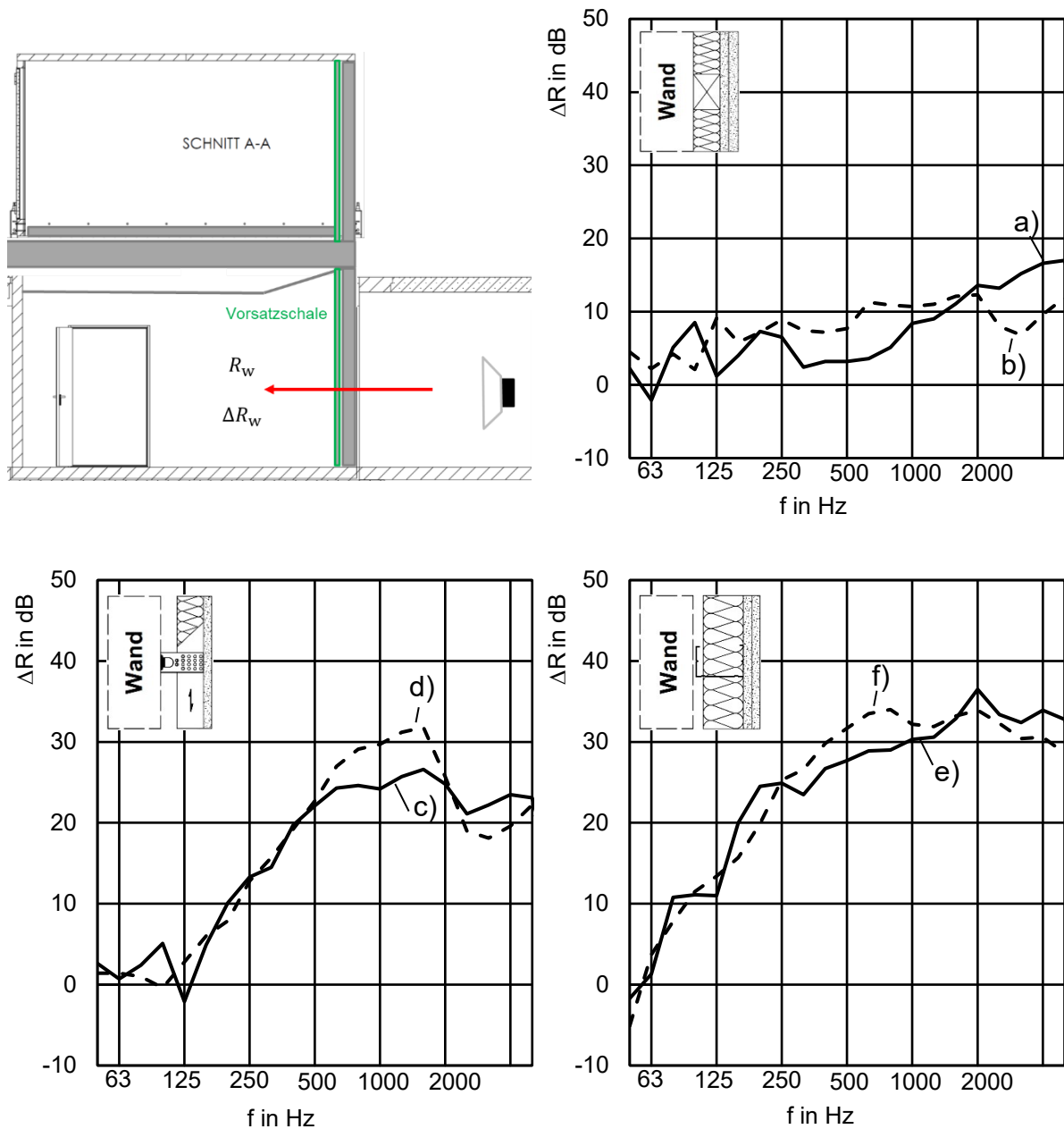
Abbildung 18 Verbesserung der Schalldämmung \Delta R von Holztafelbauwänden (HTW) und Massivholzwänden (CLT) durch unterschiedliche Vorsatzschalen (Maße in mm):
