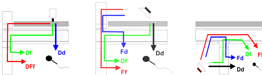
Abbildung 1 Schematische Darstellung der Beiträge zur Schallübertragung im Holzbau. Bild links: Trittschallübertragung; Bild mittig und rechts: Vertikale und horizontale Luftschallübertragung.
