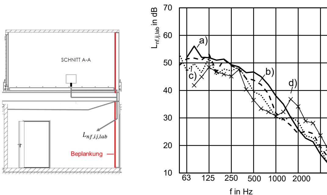
Abbildung 7 Norm-Trittschallpegel flankierender Bauteile L_{nf,ij,lab} für eine Massivholzdecke mit 60 mm Splitt und Zementestrich auf 30 mm Mineralfaser-Trittschalldämmplatten. Flankierende Massivholzwand (80 mm CLT) mit unterschiedlichen Beplankungen. Bezugsgrößen: |S_{i,ab}| = |I_{ij,lab}|
