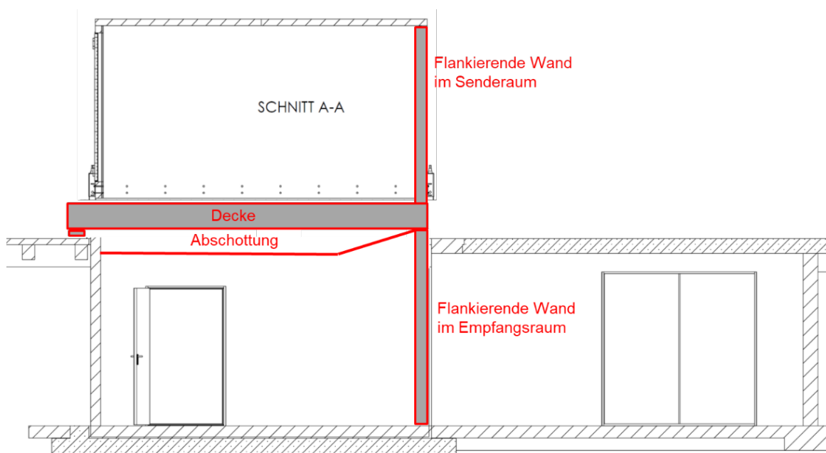
Abbildung 3 Skizze des kombinierten Wand- und Deckenprüfstandes, der für die Messungen der flankierenden Wände verwendet wurde; dargestellt für die Messung der Flankenübertragung mit hochschalldämmender Unterdecke zur Abschottung der Decke (Senderraumvolumen V_S = 52,7 \text{ m}^3 , Empfangsraumvolumen V_E = 58,8 \text{ m}^3 bzw. 65,2 \text{ m}^3 (mit bzw. ohne Unterdecke); Trennfläche S_{i,lab} = 20 \text{ m}^2 )
