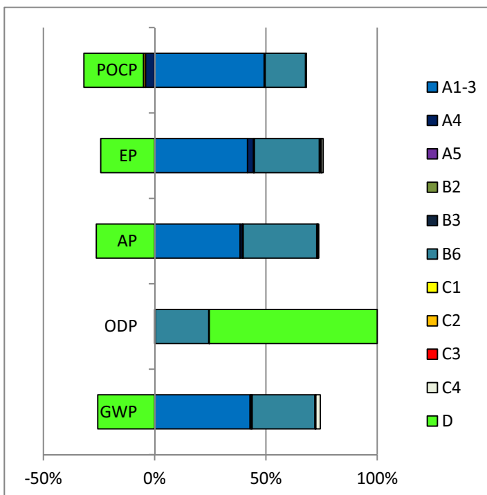
Abbildung 6: Umweltwirkungen Rolltore
