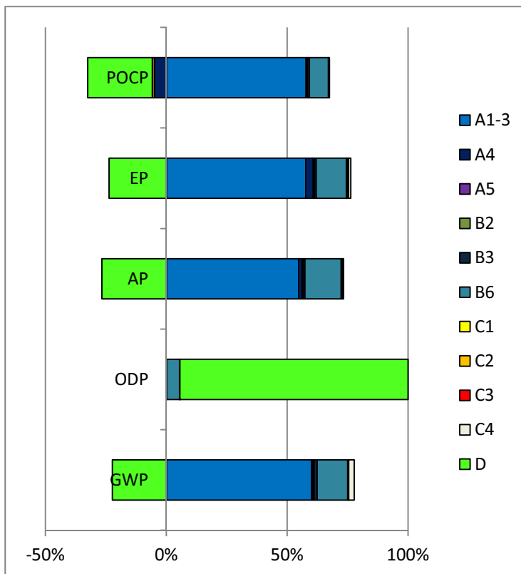
Abbildung 4: Umweltwirkungen Garagensectionaltore
